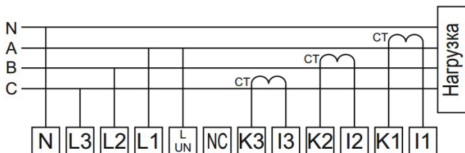
Рис. 4 – Схема подключения
