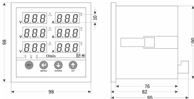
Рис. 3 – Размеры прибора
